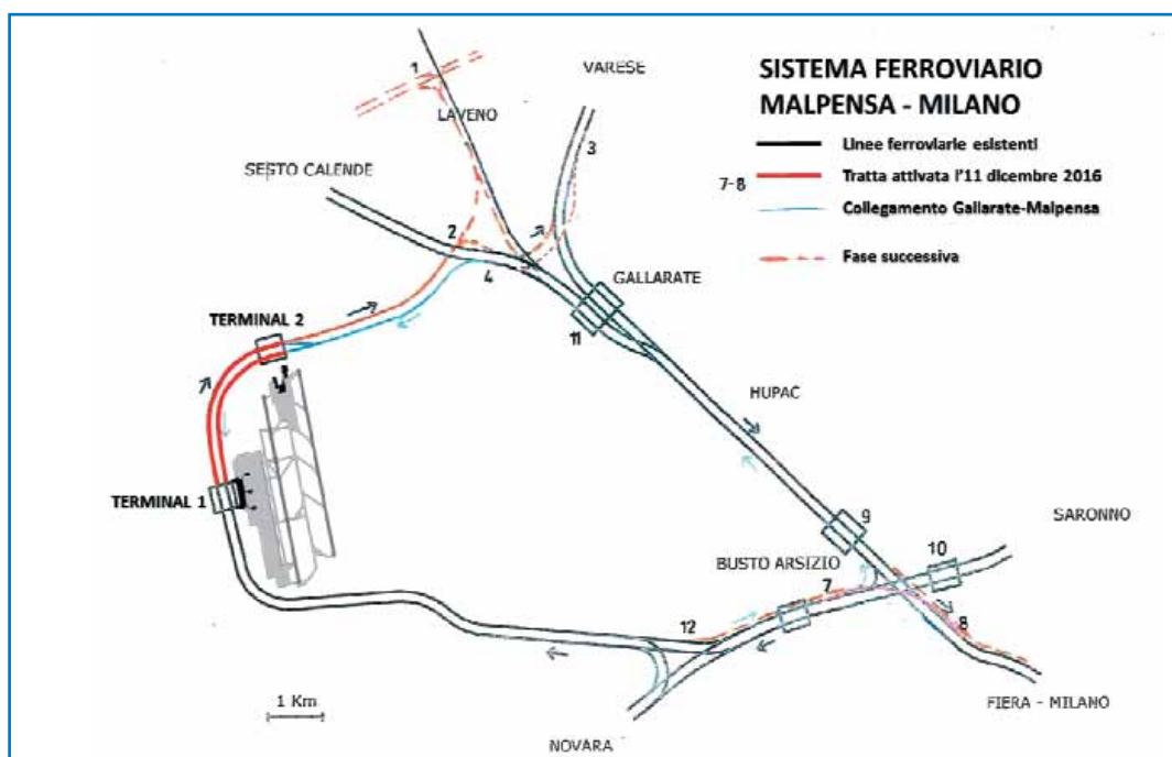
Fig. 1 – Schema delle linee ferroviarie circostanti l'aeroporto di Milano Malpensa
